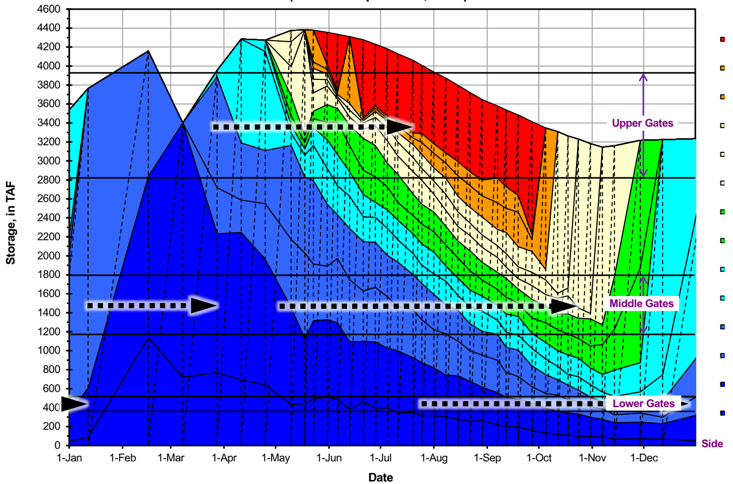
Lake Shasta Isothermobaths - 2017 (Water Temperature, in °F)
