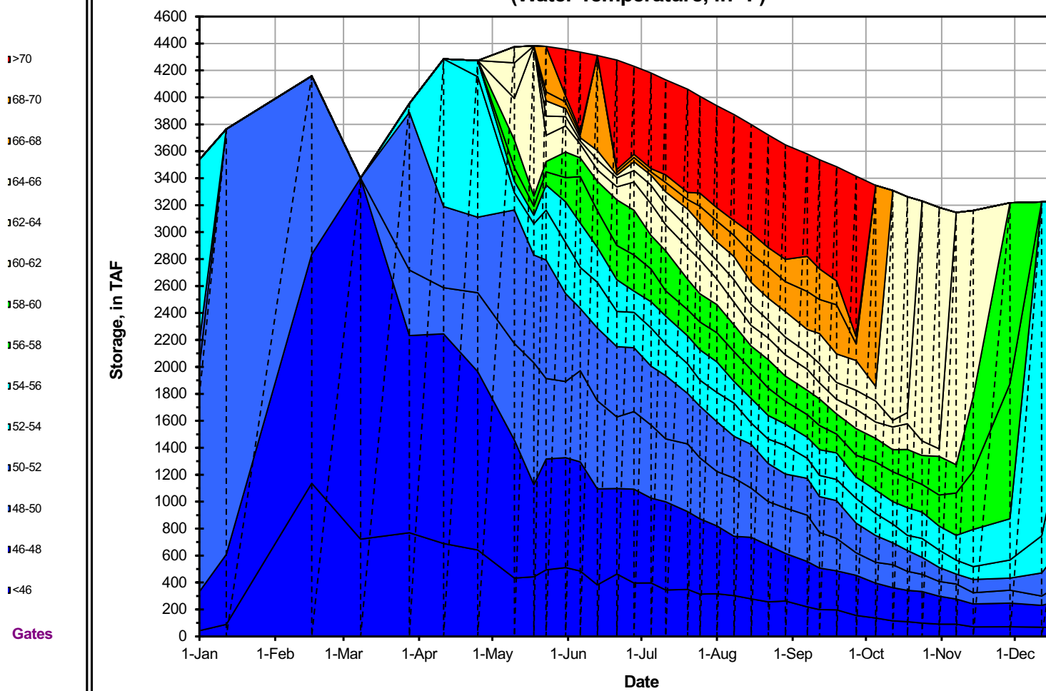
Lake Shasta Isothermobaths - 2017
